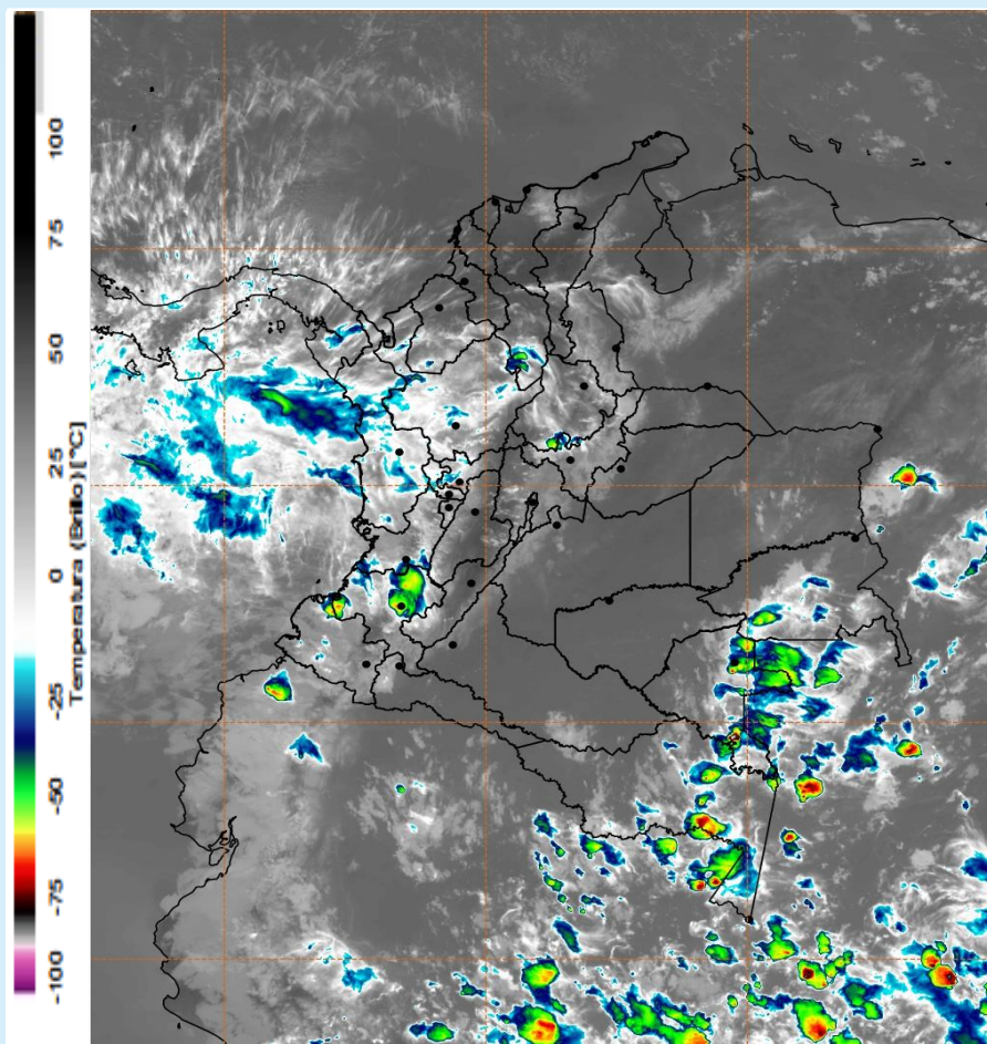
Imagen GOES 16 (East) Canal Infrarrojo 1 de febrero de 2025 - Hora 17:20 HLC Fuente: IDEAM
