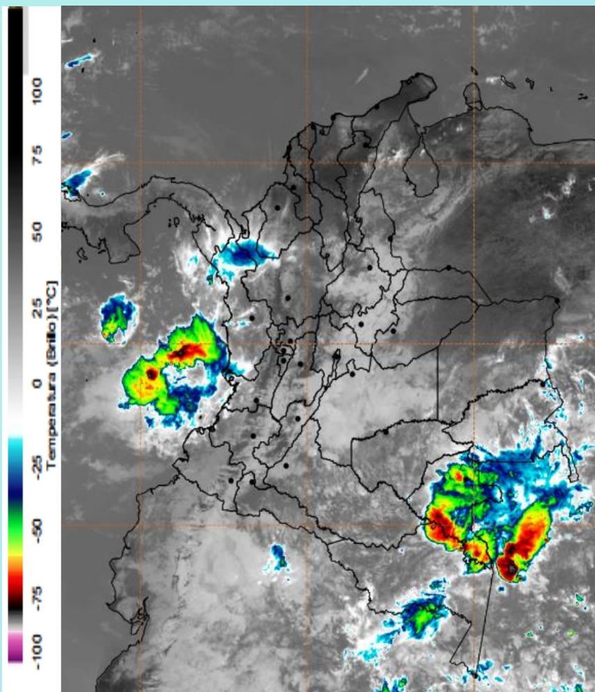
Imagen GOES East Canal Infrarrojo, 31 de enero de 2025 - Hora 11:40 HLC. Fuente: GOES 16
