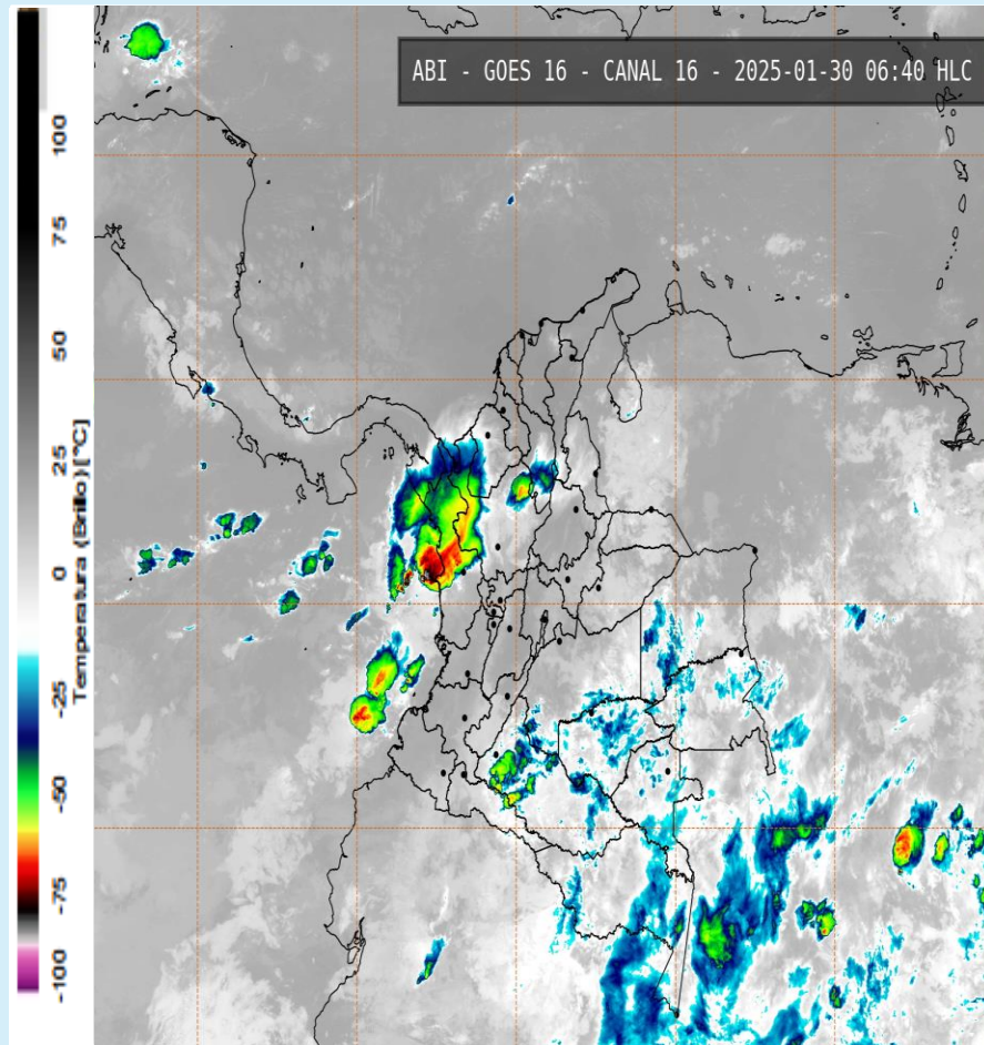
Imagen GOES 16 (East) Canal Infrarrojo 30 de enero de 2025 - Hora 06:40 HLC Fuente: IDEAM
