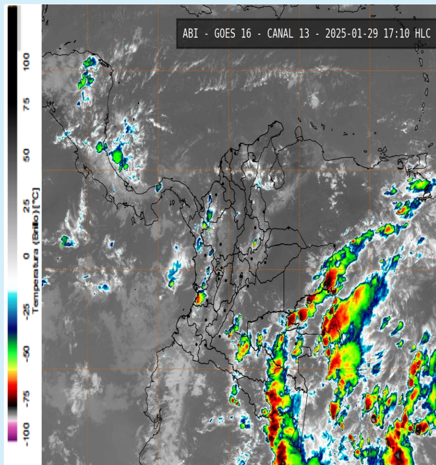
Imagen GOES 16 (East) Canal Infrarrojo 29 de enero de 2025 - Hora 17:10 HLC Fuente: IDEAM
