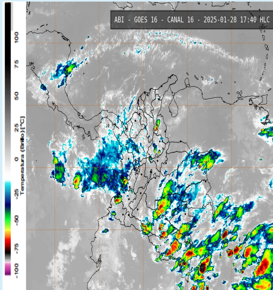
Imagen GOES 16 (East) Canal Infrarrojo 28 de enero de 2025 - Hora 17:40 HLC Fuente: IDEAM
