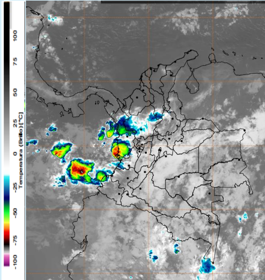
Imagen GOES 16 (East) Canal Infrarrojo 27 de enero de 2025 - Hora 06:50 HLC Fuente: IDEAM
