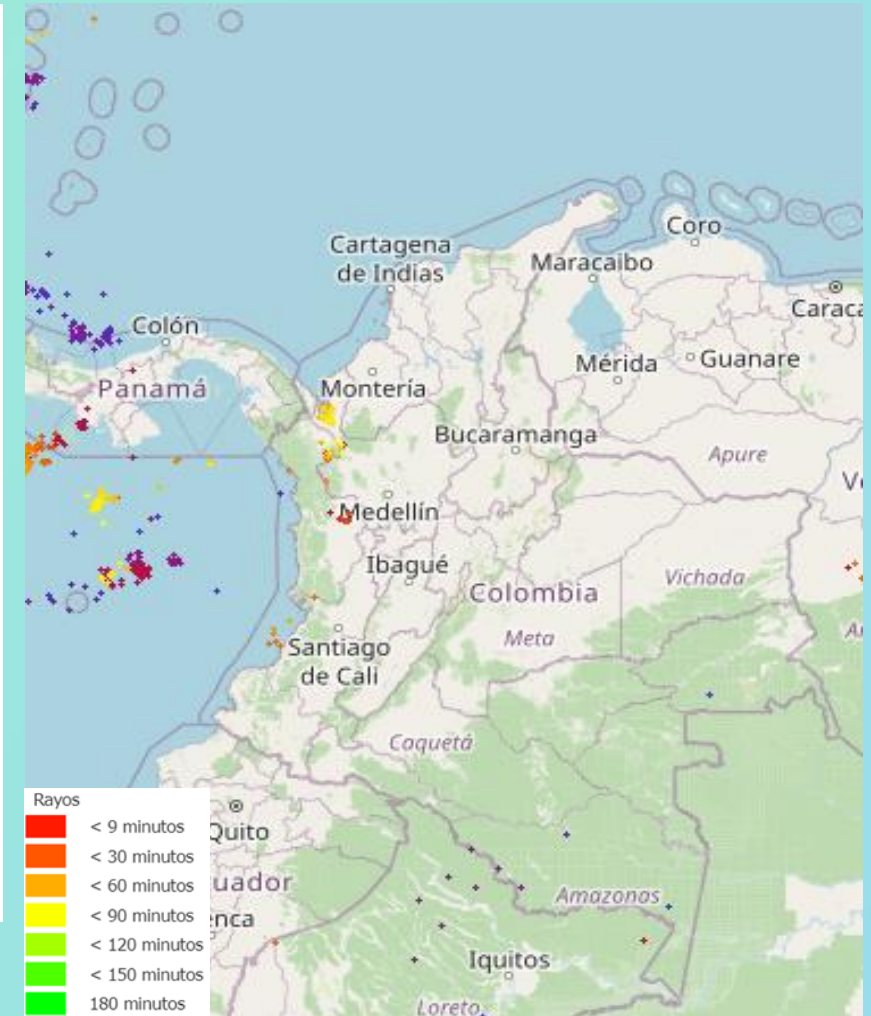
Descargas eléctricas en la última hora. Fuente: lightningmaps.org
