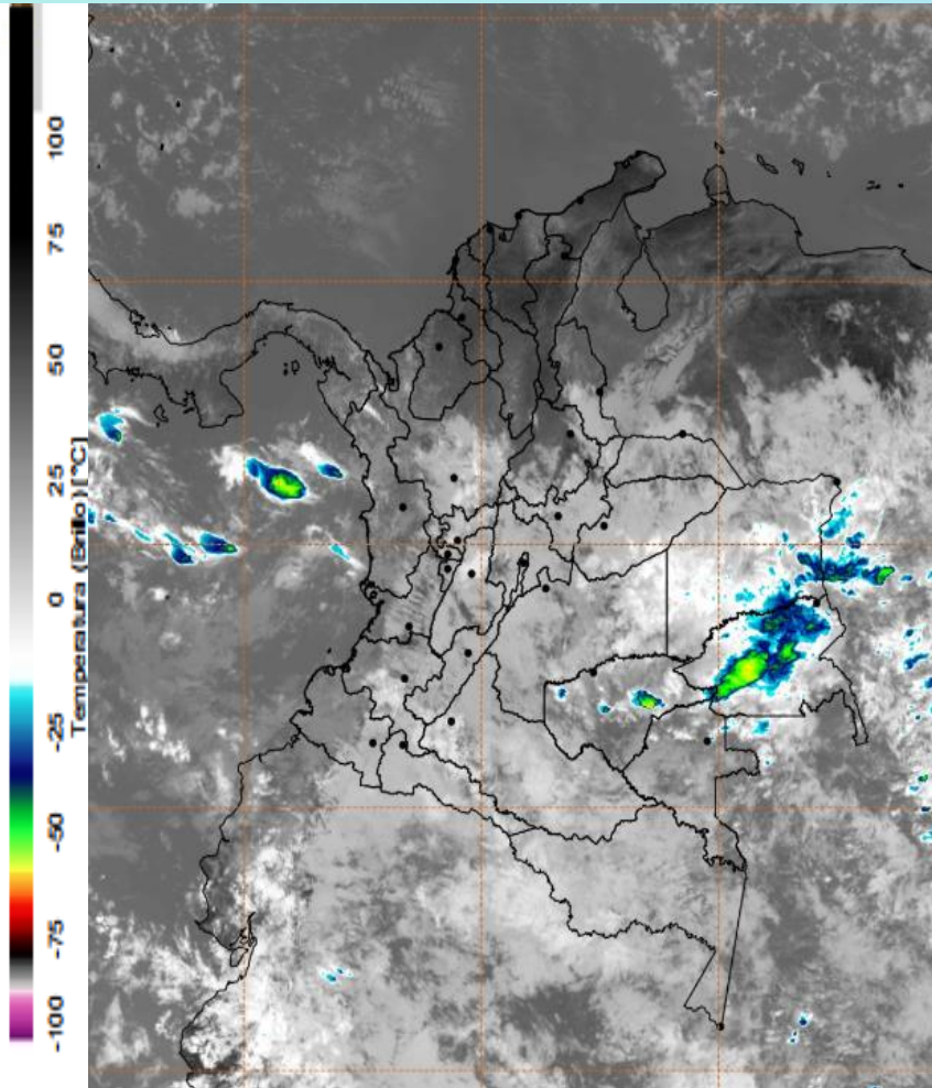
Imagen GOES East Canal Infrarrojo, 24 de enero de 2025 - Hora 11:50 HLC. Fuente: GOES 16
