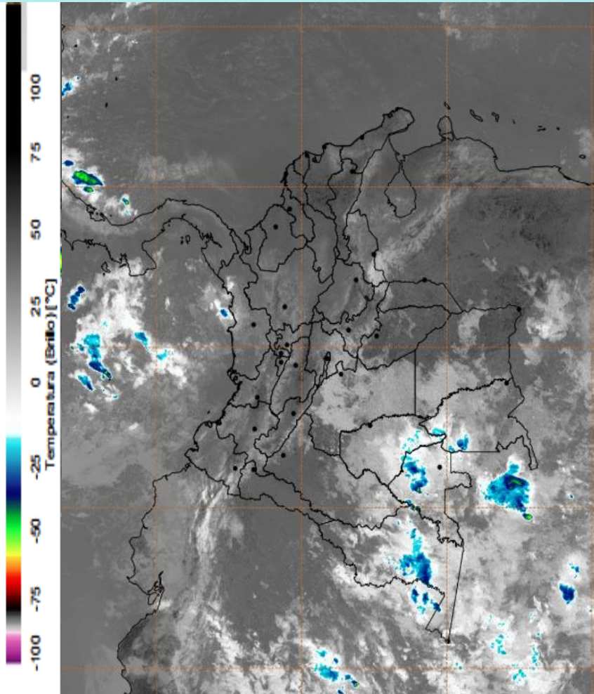
Imagen GOES East Canal Infrarrojo, 23 de enero de 2025 - Hora 11:50 HLC. Fuente: GOES 16
