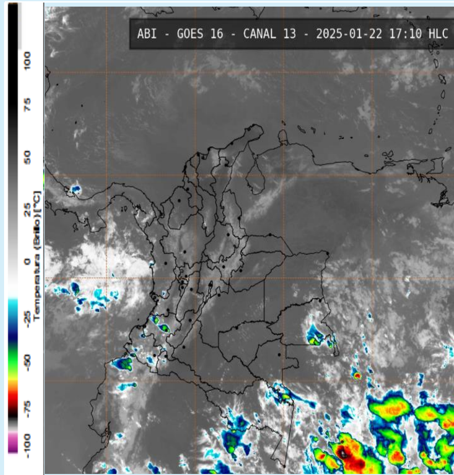
Imagen GOES 16 (East) Canal Infrarrojo 22 de enero de 2025 - Hora 17:10 HLC Fuente: IDEAM
