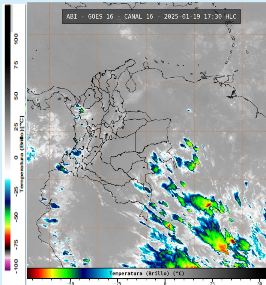
Imagen GOES 16 (East) Canal Infrarrojo 19 de enero de 2025 - Hora 17:30 HLC Fuente: IDEAM
