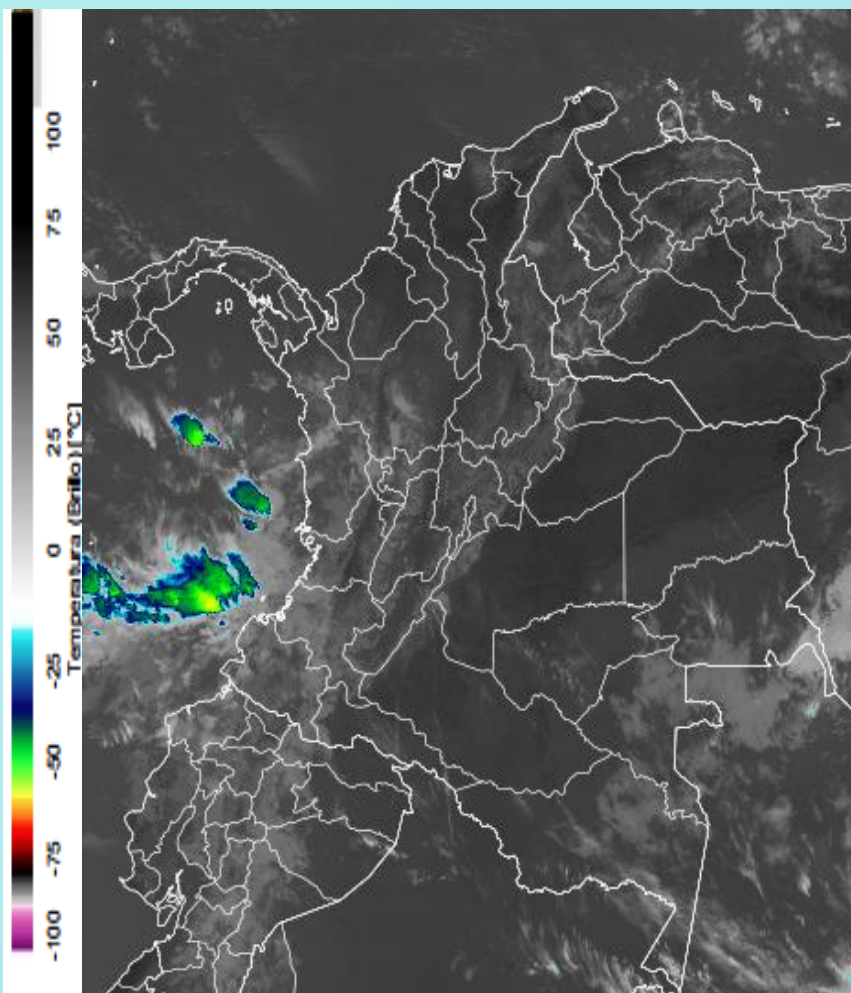
Imagen GOES East Canal Infrarrojo, 19 de enero de 2025 - Hora 11:40 HLC. Fuente: GOES 16
