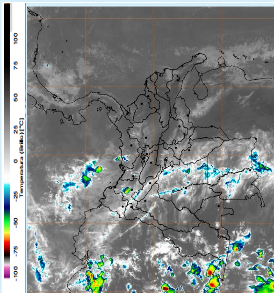
Imagen GOES 16 (East) Canal Infrarrojo 14 de enero de 2025 - Hora 17:30 HLC Fuente: CIRA
