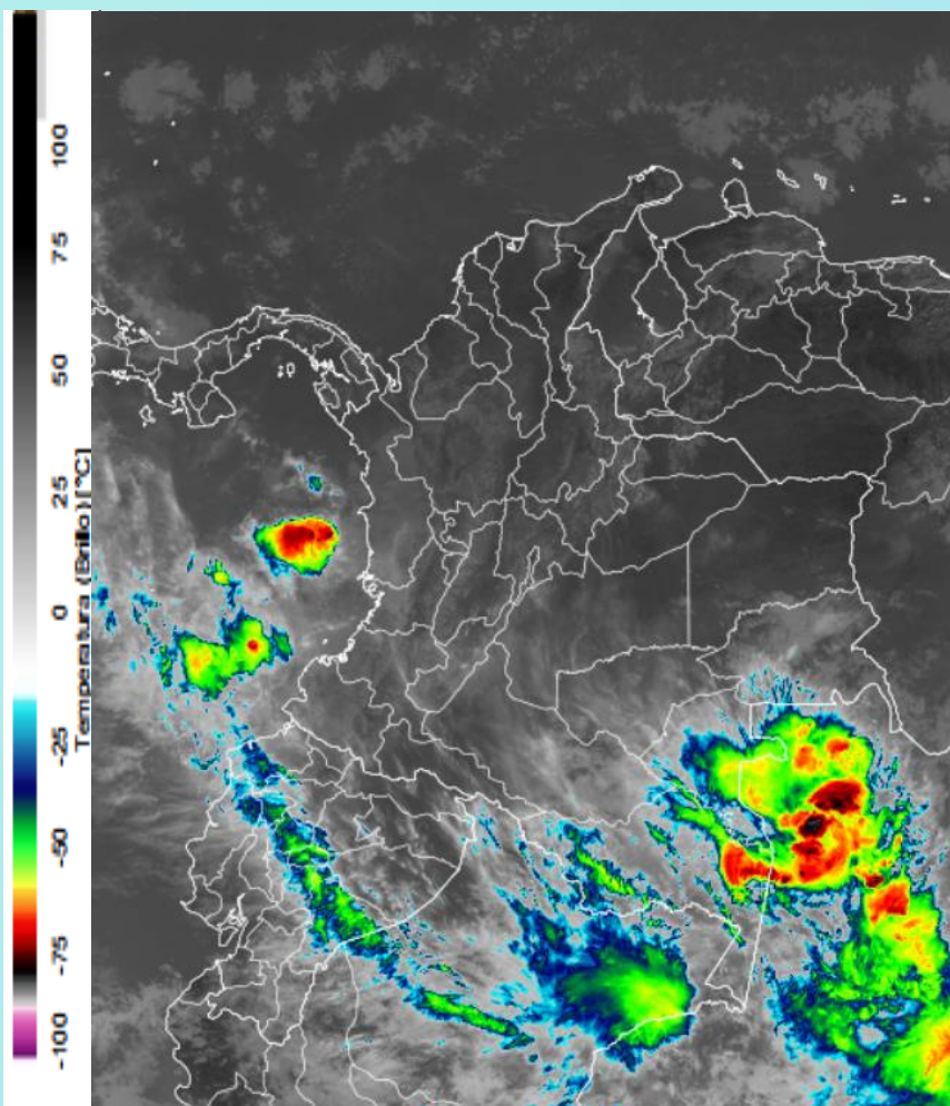
Imagen GOES East Canal Infrarrojo, 13 de enero de 2025 - Hora 12:00 HLC. Fuente: GOES 16
