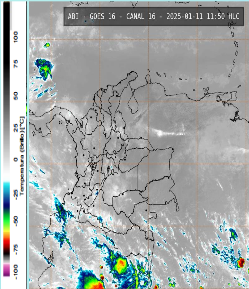
Imagen GOES East Canal Infrarrojo, 11 de enero de 2025 - Hora 11:50 HLC. Fuente: GOES 16
