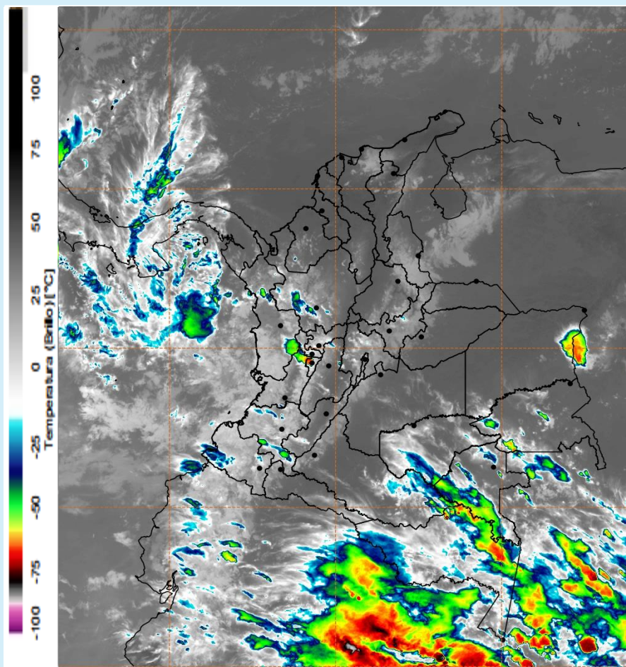
Imagen GOES 16 (East) Canal Infrarrojo 9 de enero de 2025 - Hora 17:20 HLC Fuente: IDEAM
