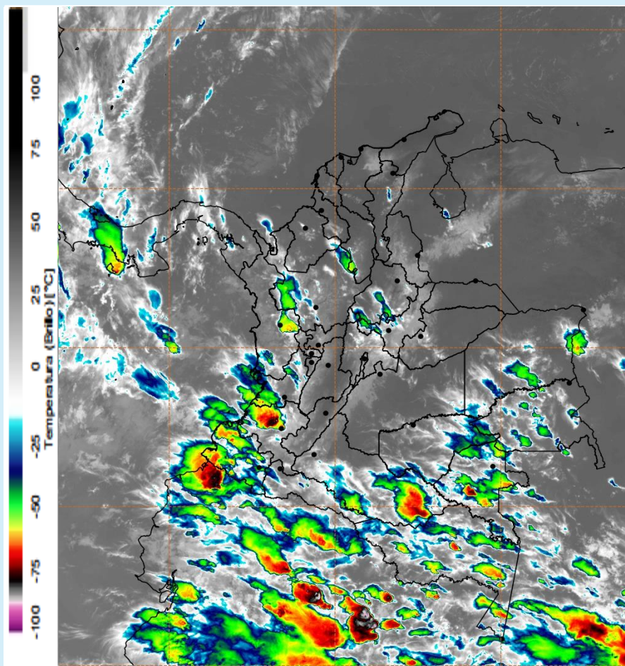
Imagen GOES 16 (East) Canal Infrarrojo 7 de enero de 2025 - Hora 17:20 HLC Fuente: IDEAM
