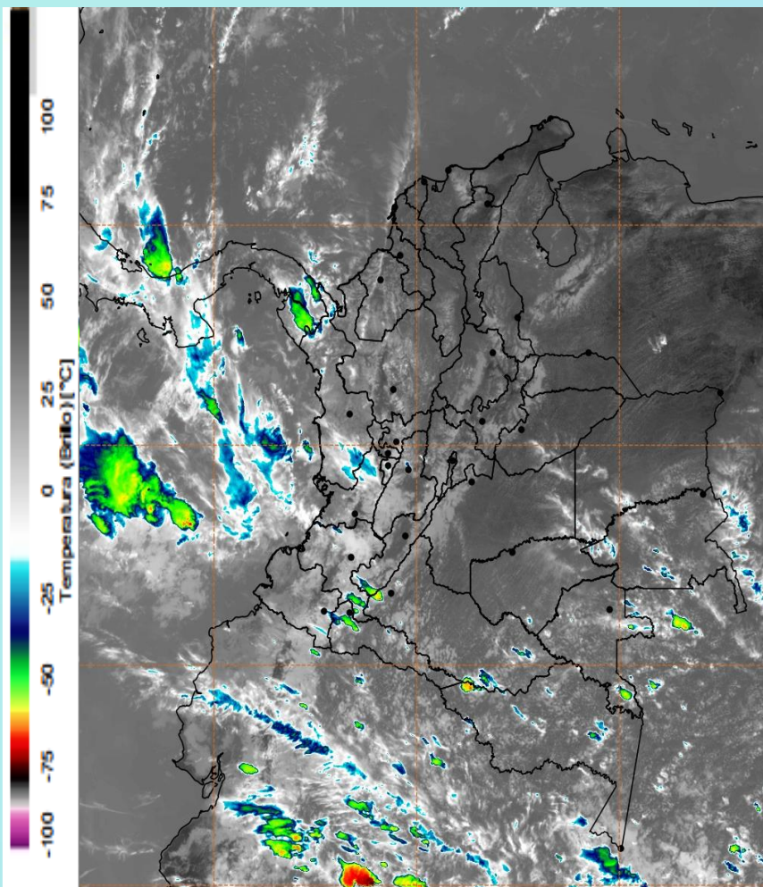
Imagen GOES East Canal Infrarrojo, 7 de enero de 2025 - Hora 12:10 HLC. Fuente: GOES 16
