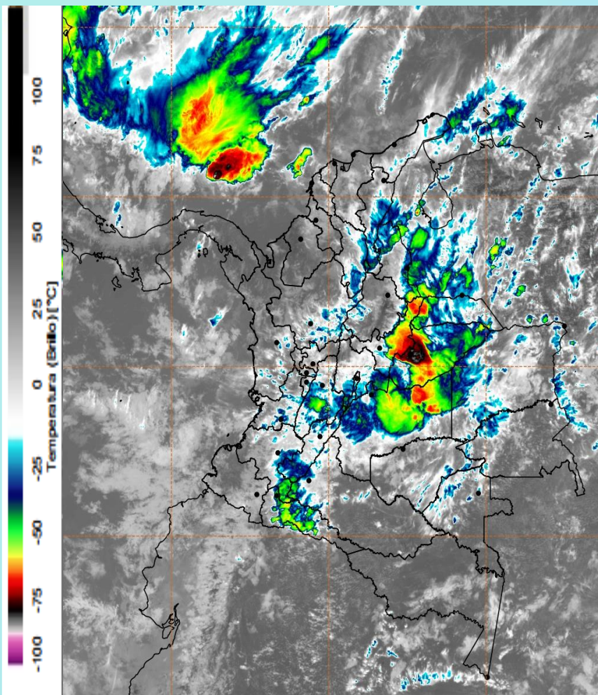
Imagen GOES East Canal Infrarrojo, 5 de enero de 2025 - Hora 12:00 HLC. Fuente: GOES 16
