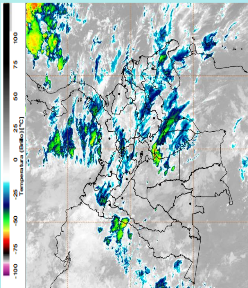
Imagen GOES East Canal Infrarrojo, 3 de enero de 2025 - Hora 11:30 HLC. Fuente: GOES 16
