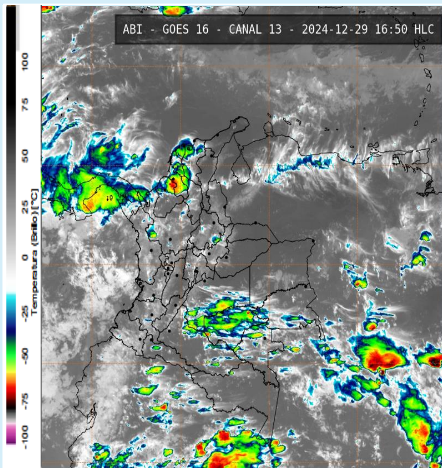
Imagen GOES 16 (East) Canal Infrarrojo 29 de diciembre de 2024 - Hora 16:50 HLC Fuente: IDEAM
