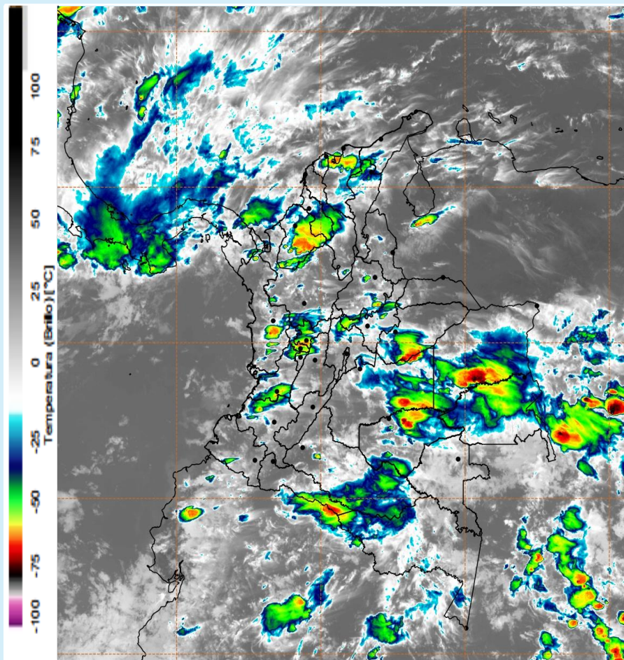
Imagen GOES 16 (East) Canal Infrarrojo 28 de diciembre de 2024 - Hora 17:10 HLC Fuente: IDEAM
