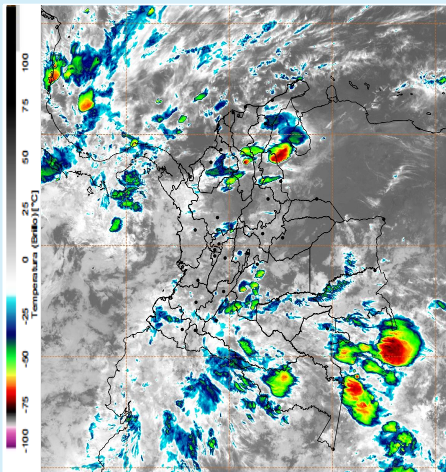
Imagen GOES 16 (East) Canal Infrarrojo 27 de diciembre de 2024 - Hora 23:10 HLC Fuente: IDEAM
