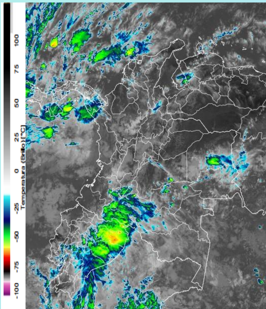
Imagen GOES East Canal Infrarrojo, 27 de diciembre de 2024 - Hora 11:40 HLC. Fuente: GOES 16
