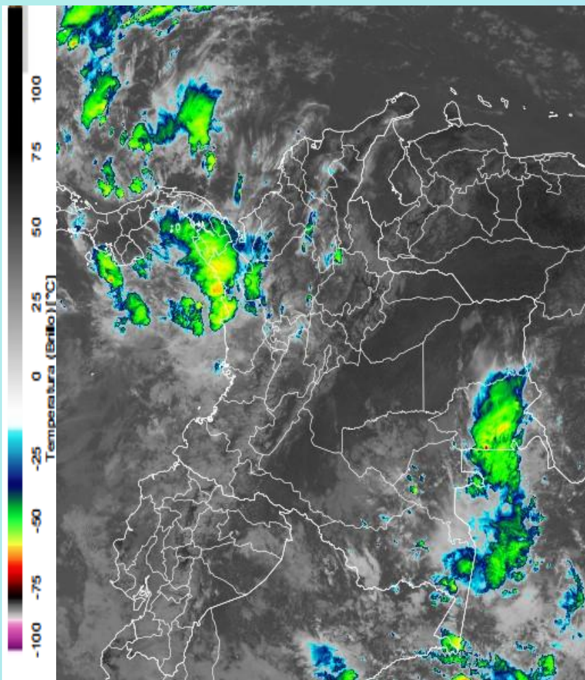
Imagen GOES East Canal Infrarrojo, 26 de diciembre de 2024 - Hora 11:40 HLC. Fuente: GOES 16
