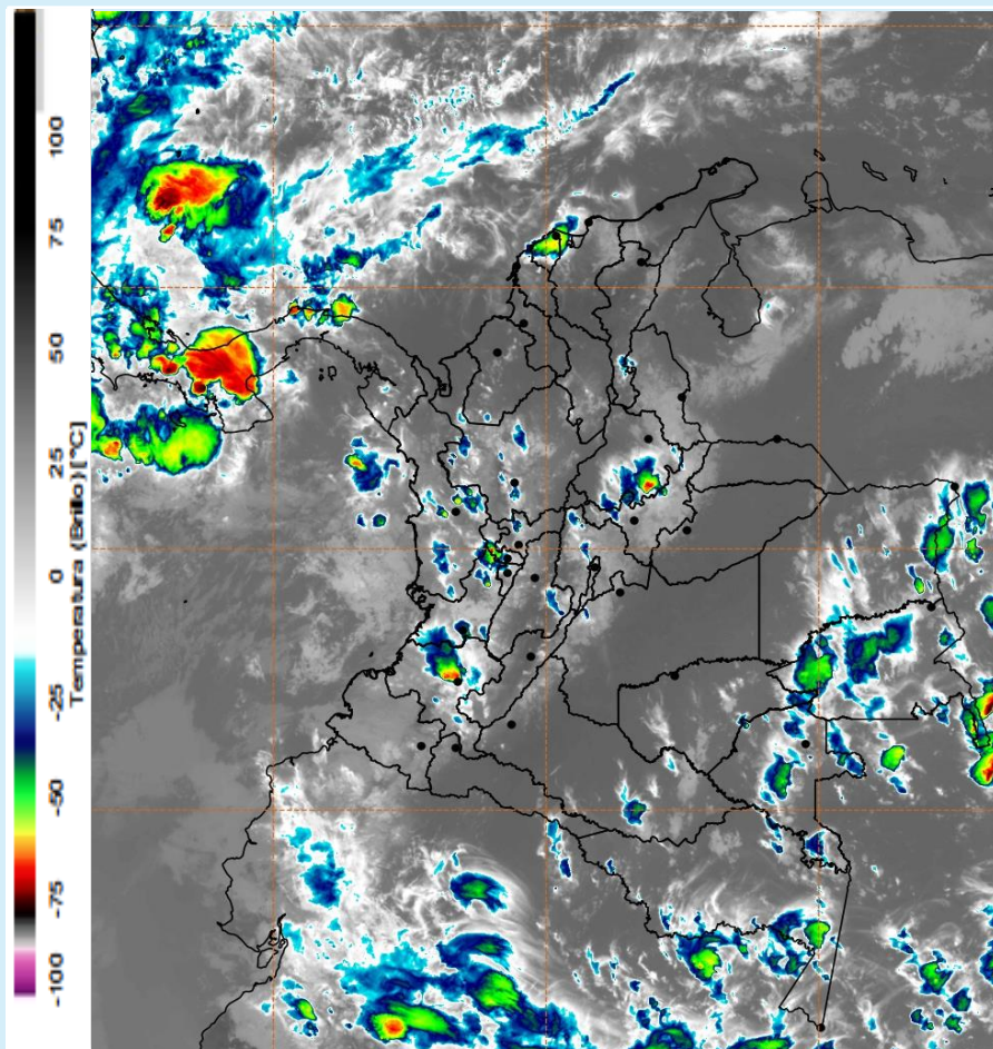
Imagen GOES 16 (East) Canal Infrarrojo 25 de diciembre de 2024 - Hora 17:10 HLC Fuente: IDEAM
