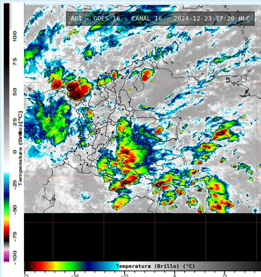
Imagen GOES 16 (East) Canal Infrarrojo | 23 de diciembre de 2024 - Hora 17:20 HLC Fuente: IDEAM
