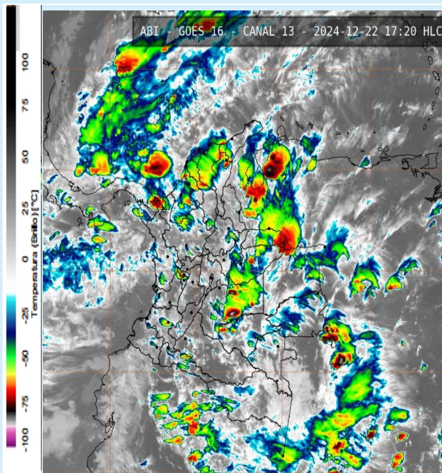
Imagen GOES 16 (East) Canal Infrarrojo | 22 de diciembre de 2024 - Hora 05:00 HLC Fuente: IDEAM
