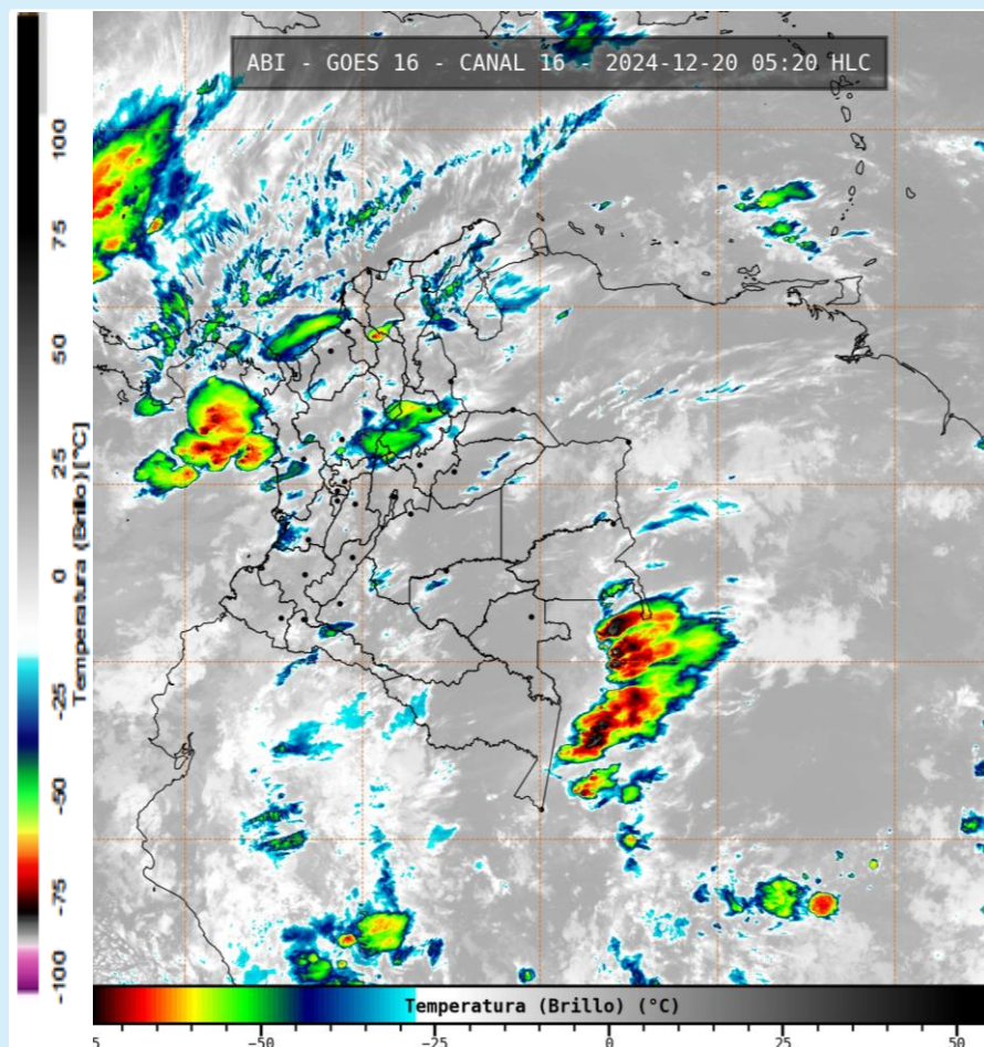
Imagen GOES 16 (East) Canal Infrarrojo | 20 de diciembre de 2024 - Hora 05:20 HLC Fuente: IDEAM
