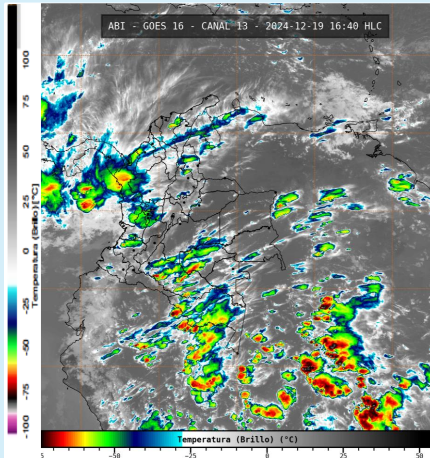
Imagen GOES 16 (East) Canal Infrarrojo | 19 de diciembre de 2024 - Hora 16:40 HLC Fuente: IDEAM
