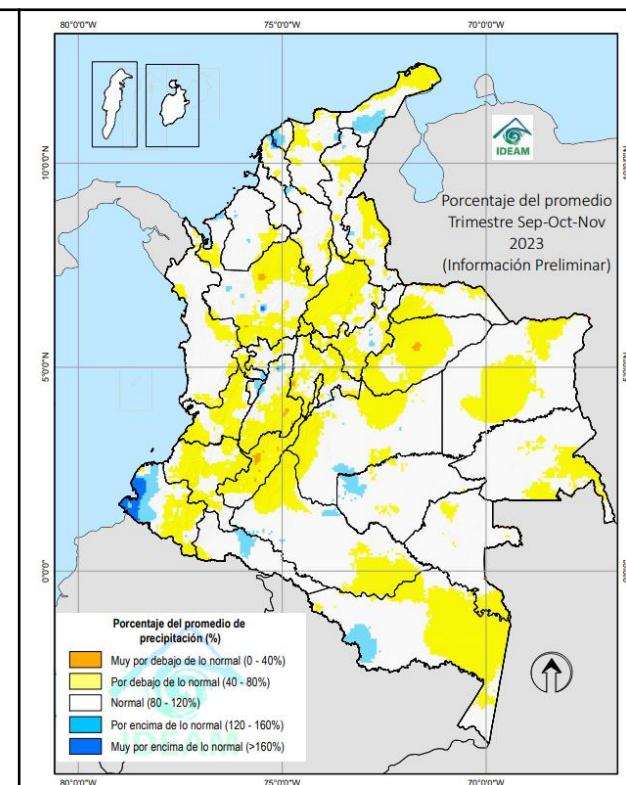
Índice Precipitación Trimestre (Sep-Oct- Nov) (%)
