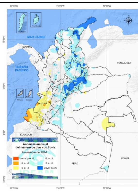
Anomalía de número de días con lluvia
