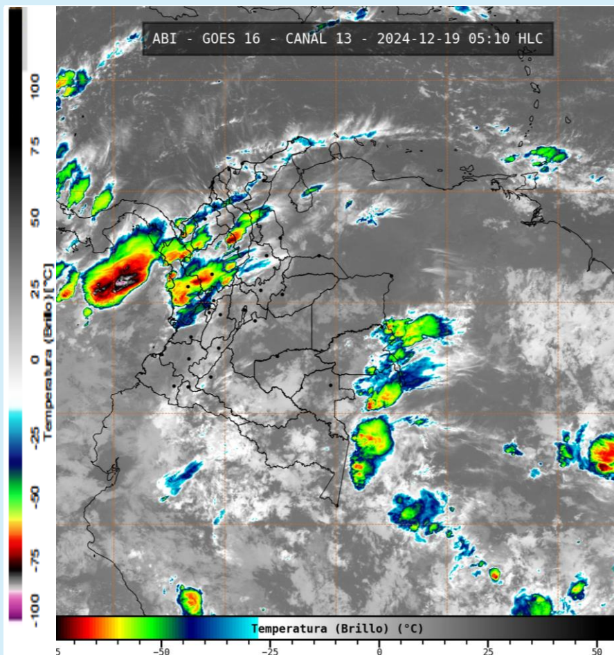
Imagen GOES 16 (East) Canal Infrarrojo | 19 de diciembre de 2024 - Hora 05:10 HLC Fuente: IDEAM
