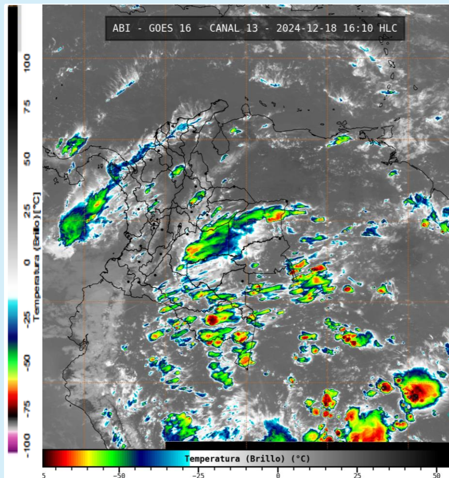
Imagen GOES 16 (East) Canal Infrarrojo | 18 de diciembre de 2024 - Hora 16:10 HLC Fuente: IDEAM
