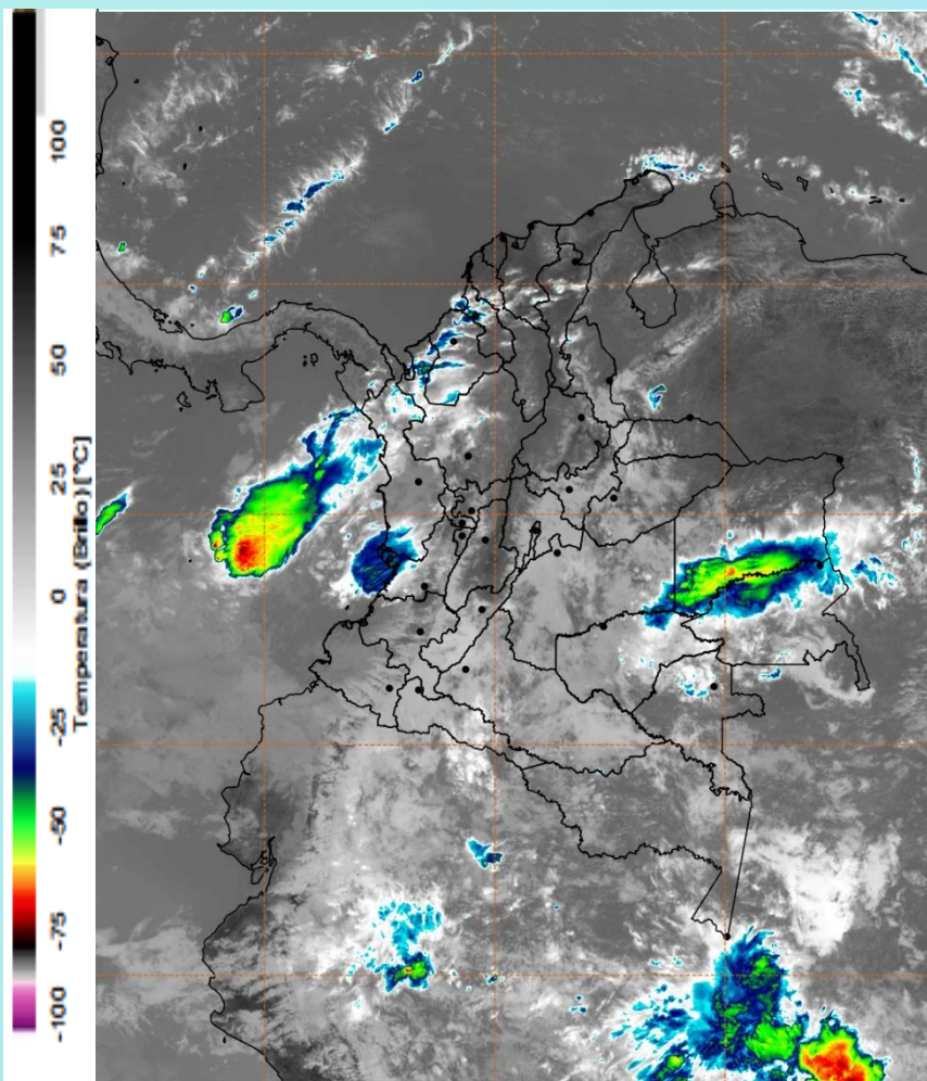
Imagen GOES East Canal Infrarrojo, 18 de diciembre de 2024 - Hora 11:10 HLC. Fuente: GOES 16
