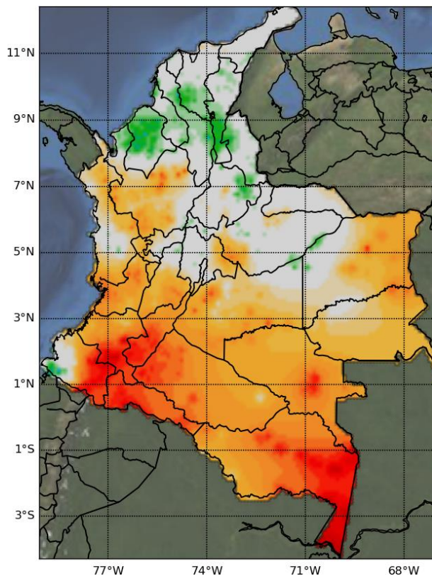
Índice estandarizado de evapotranspiración a: 06 meses Periodo: 11-2023
