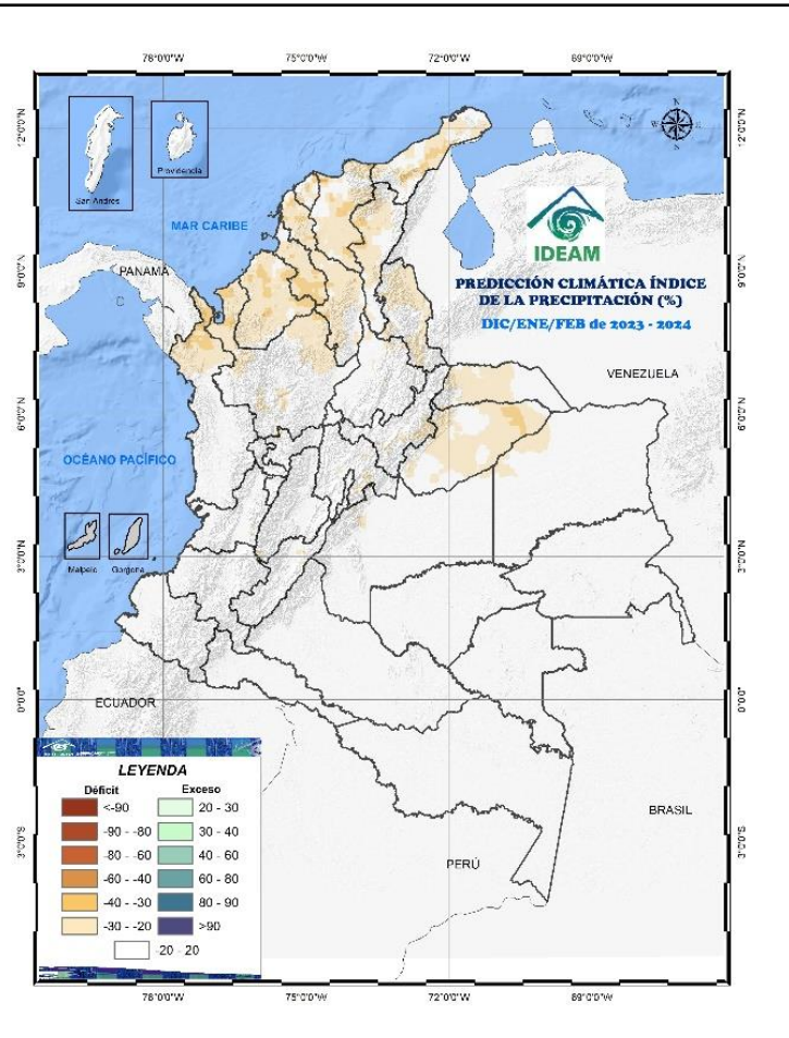
Cambio de la Precipitación (%)
