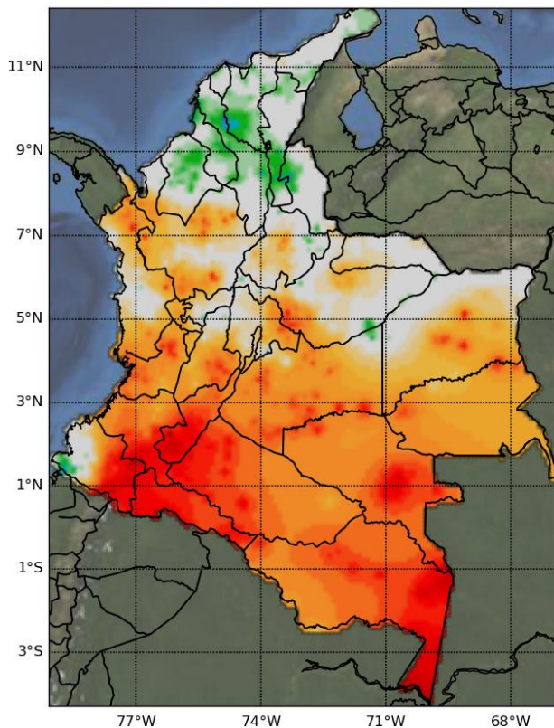
Índice estandarizado de evapotranspiración a: 03 meses Periodo: 11-2023
