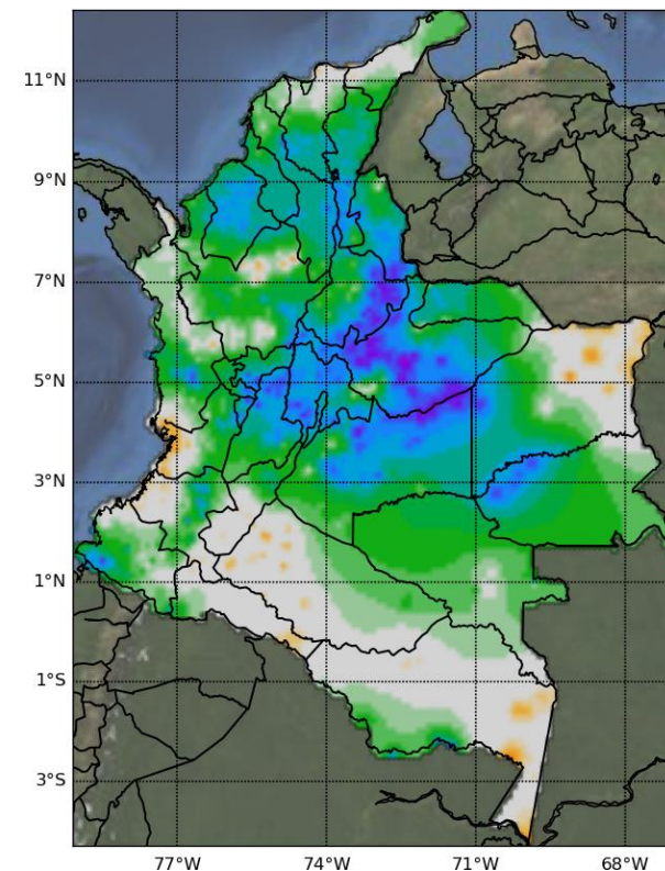
Índice estandarizado de evapotranspiración a: 12 meses Periodo: 11-2023
