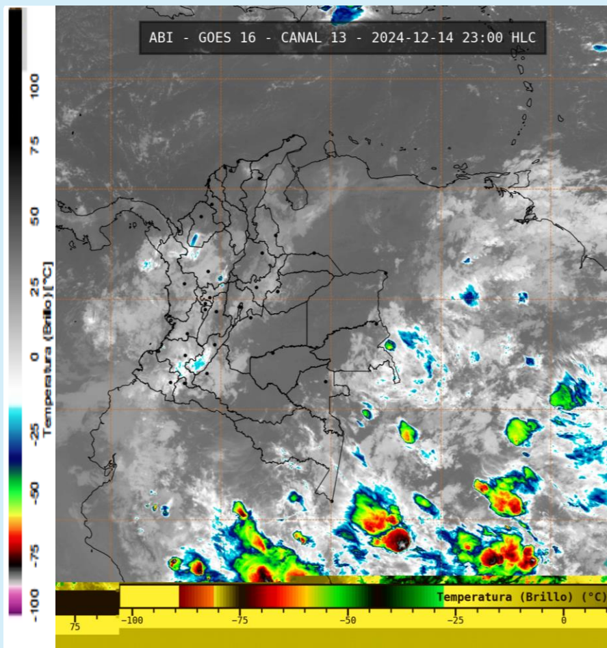
Imagen GOES 16 (East) Canal Infrarrojo | 14 de diciembre de 2024 - Hora 22:40 HLC Fuente: IDEAM
