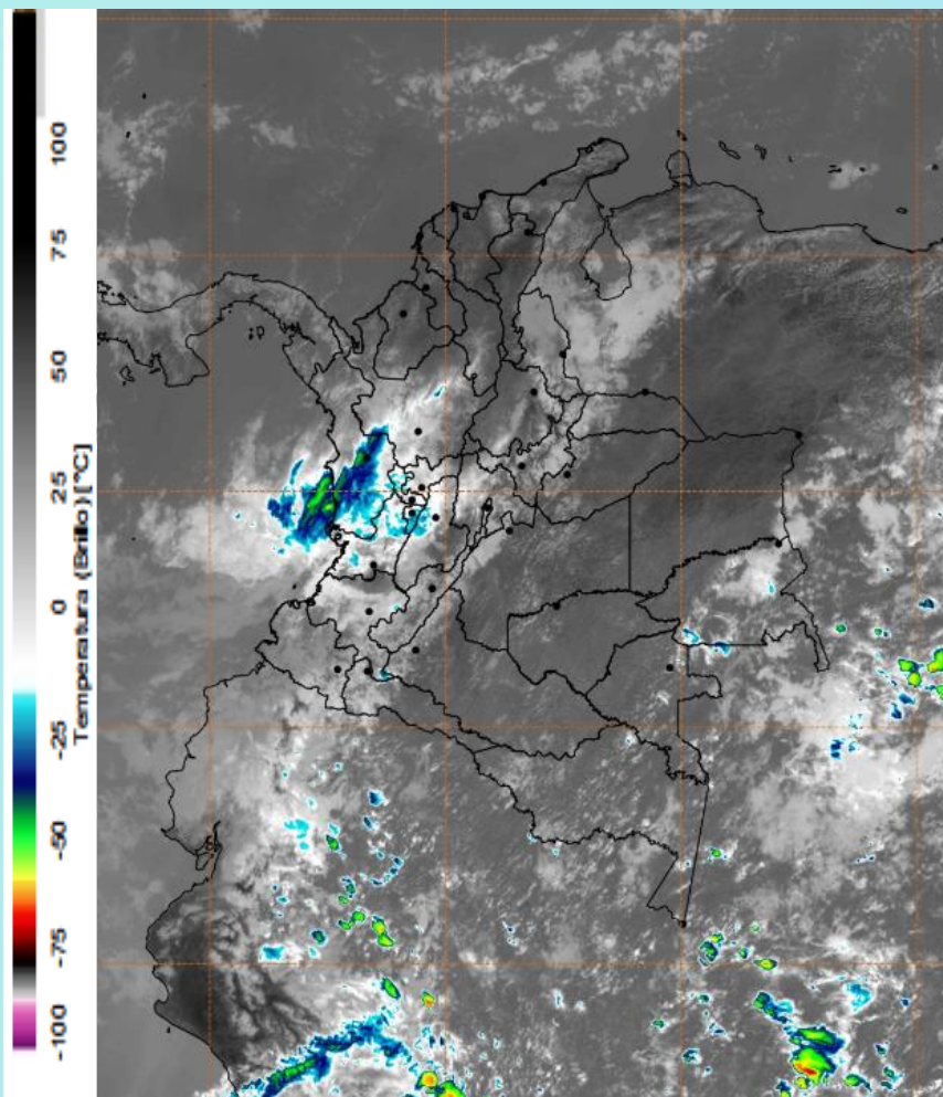
Imagen GOES East Canal Infrarrojo, 14 de diciembre de 2024 - Hora 11:50 HLC. Fuente: GOES 16
