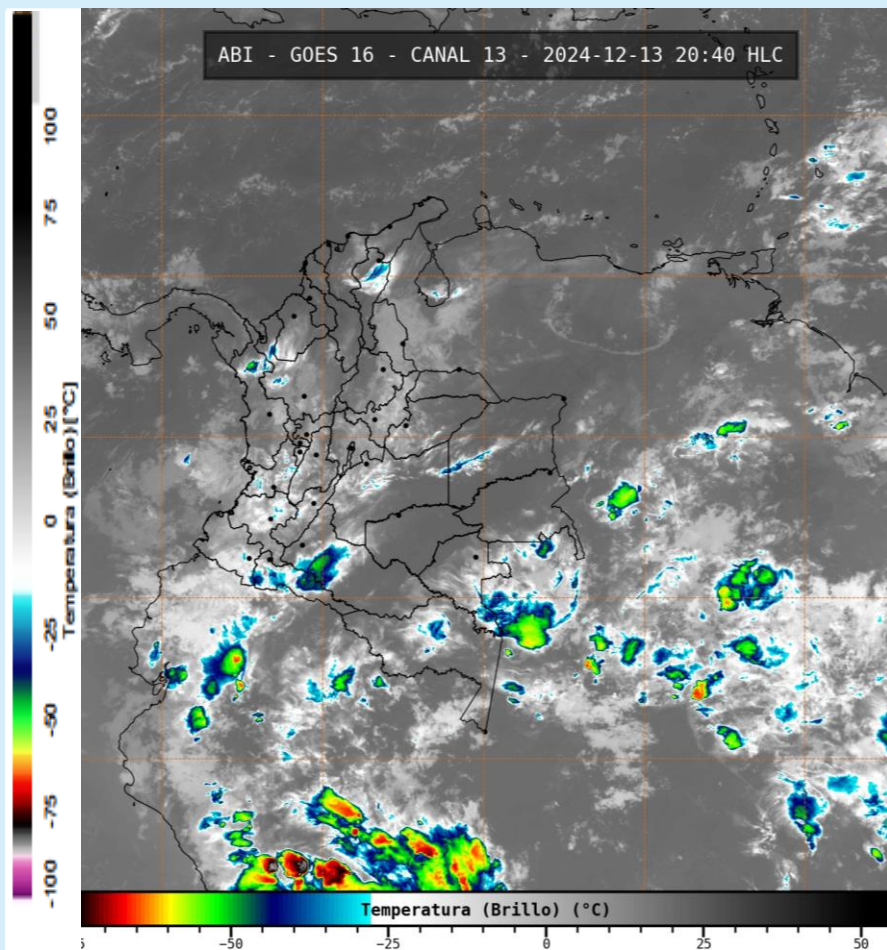
Imagen GOES 16 (East) Canal Infrarrojo | 13 de diciembre de 2024 - Hora 23:00 HLC Fuente: IDEAM
