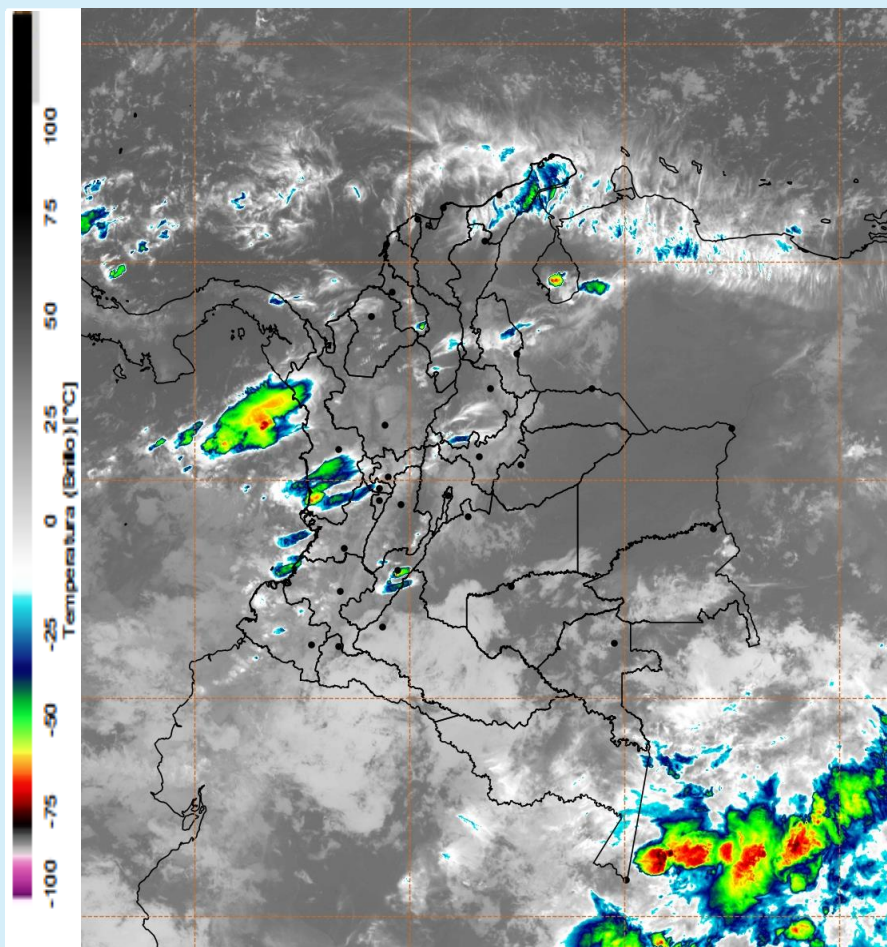
Imagen GOES 16 (East) Canal Infrarrojo | 12 de diciembre de 2024 - Hora 05:00 HLC Fuente: IDEAM
