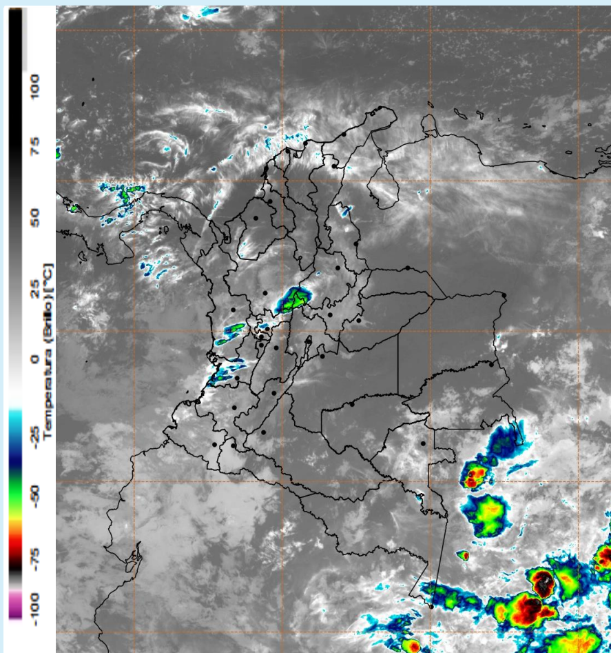
Imagen GOES 16 (East) Canal Infrarrojo | 11 de diciembre de 2024 - Hora 23:10 HLC Fuente: IDEAM
