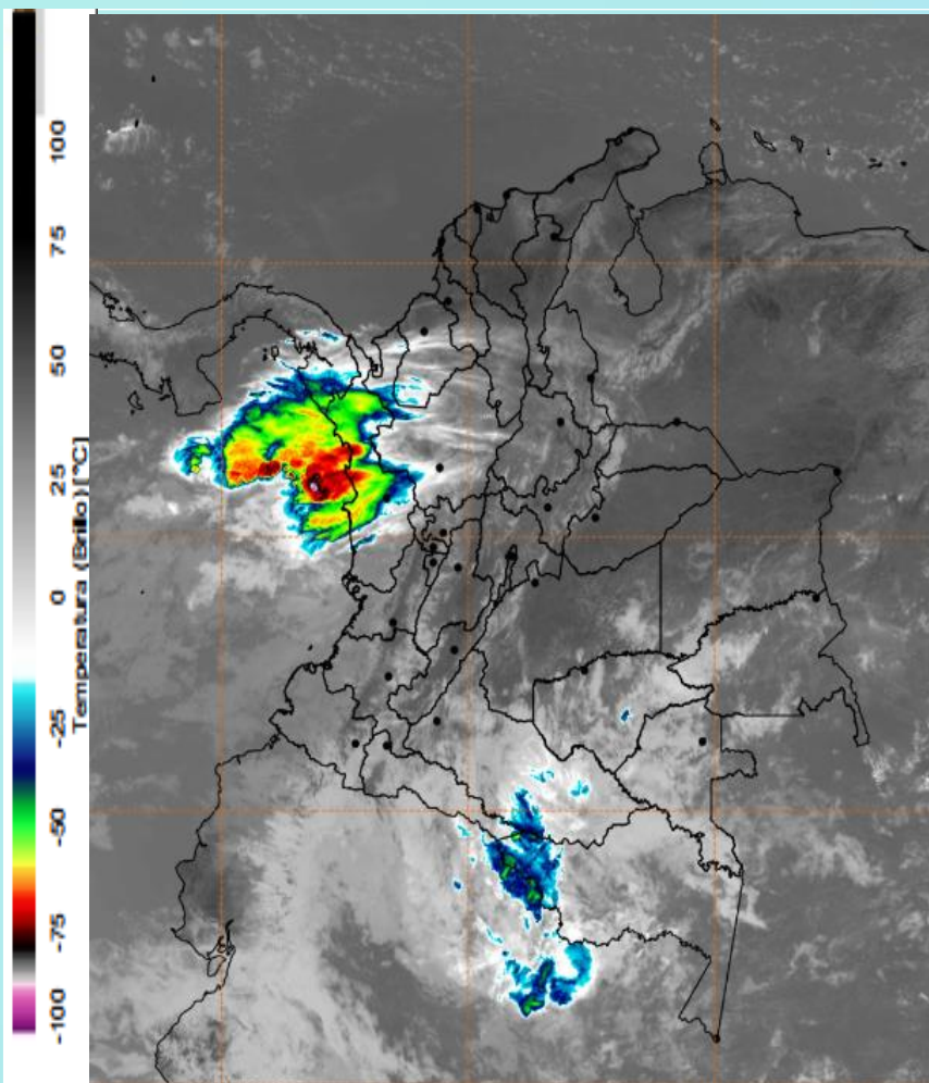
Imagen GOES East Canal Infrarrojo, 11 de diciembre de 2024 - Hora 10:30 HLC. Fuente: GOES 16
