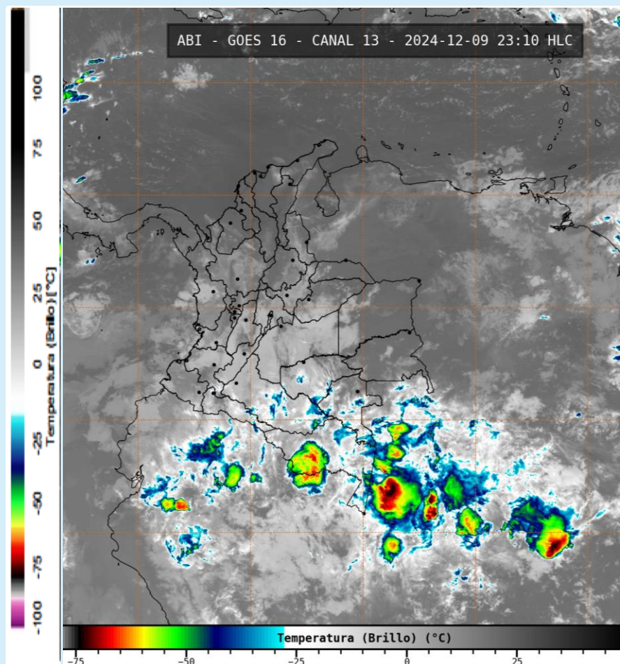
Imagen GOES 16 (East) Canal Infrarrojo | 9 de diciembre de 2024 - Hora 23:10 HLC Fuente: IDEAM
