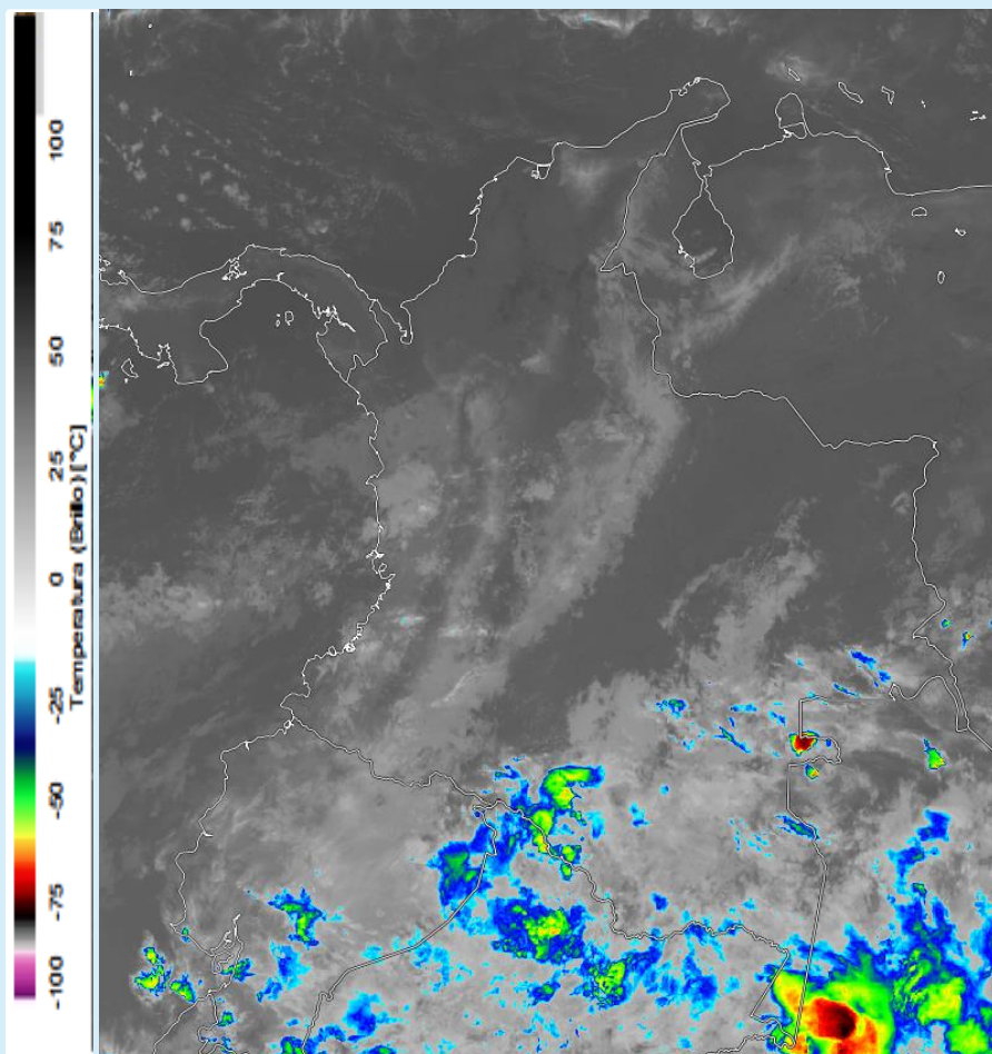
Imagen GOES 16 (East) Canal Infrarrojo | 8 de diciembre de 2024 - Hora 23:20 HLC
