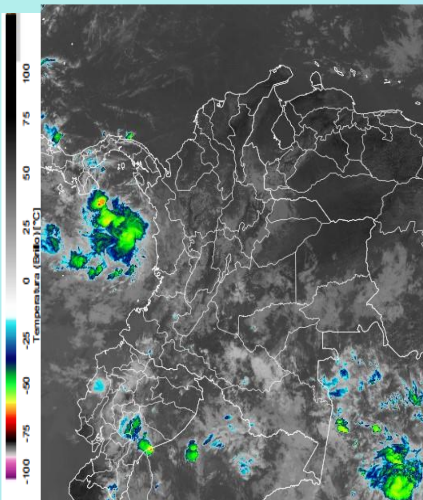
Imagen GOES East Canal Infrarrojo, 6 de diciembre de 2024 - Hora 11:40 HLC. Fuente: GOES 16
