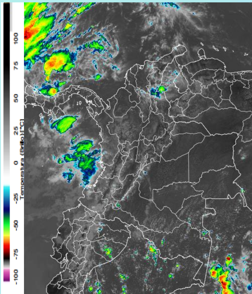
Imagen GOES East Canal Infrarrojo, 3 de diciembre de 2024 - Hora 12:00 HLC. Fuente: GOES 16
