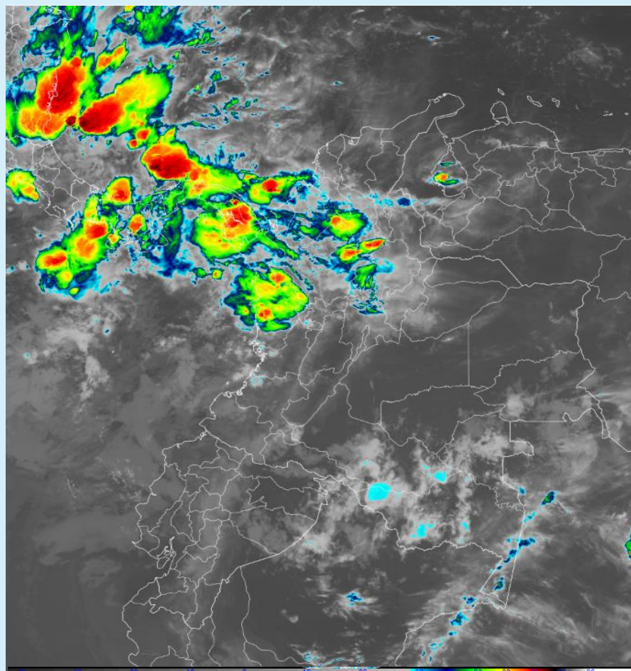
Imagen GOES 16 (East) Canal Infrarrojo | 2 de diciembre de 2024 - Hora 05:50 HLC
