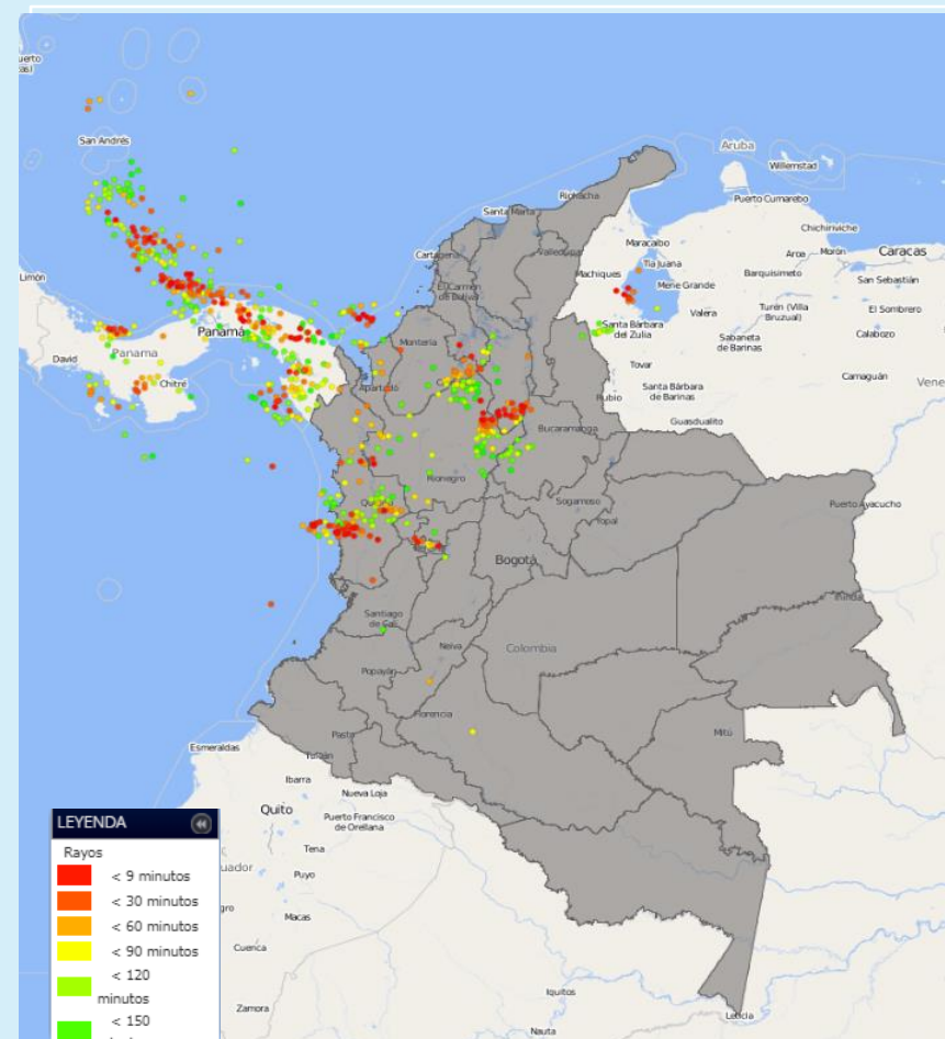
Descargas eléctricas en las últimas 3 horas
