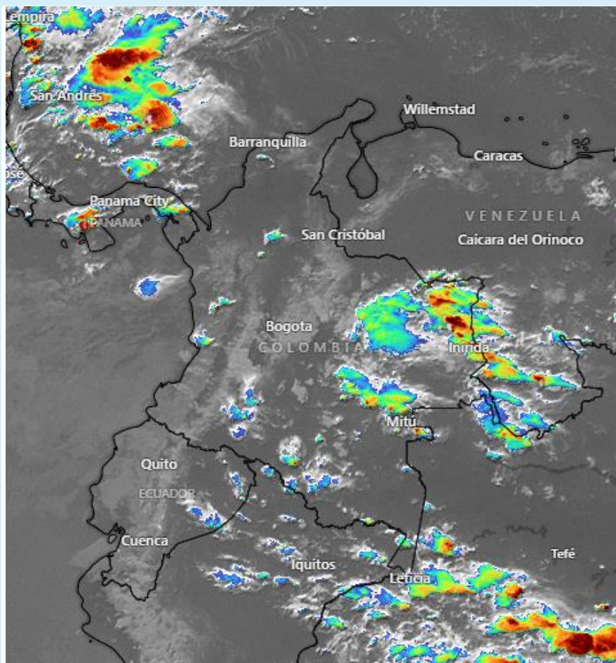
Imagen GOES 16 (East) Canal Infrarrojo | 30 de noviembre de 2024 - Hora 15:30 HLC Fuente: https://rammb-slider.cira.colostate.edu/
