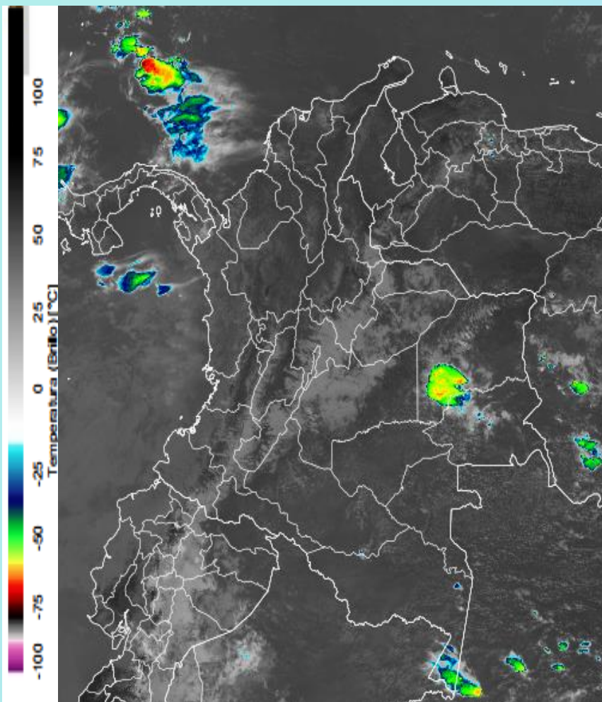
Imagen GOES East Canal Infrarrojo, 30 de noviembre de 2024 - Hora 12:00 HLC. Fuente: GOES 16
