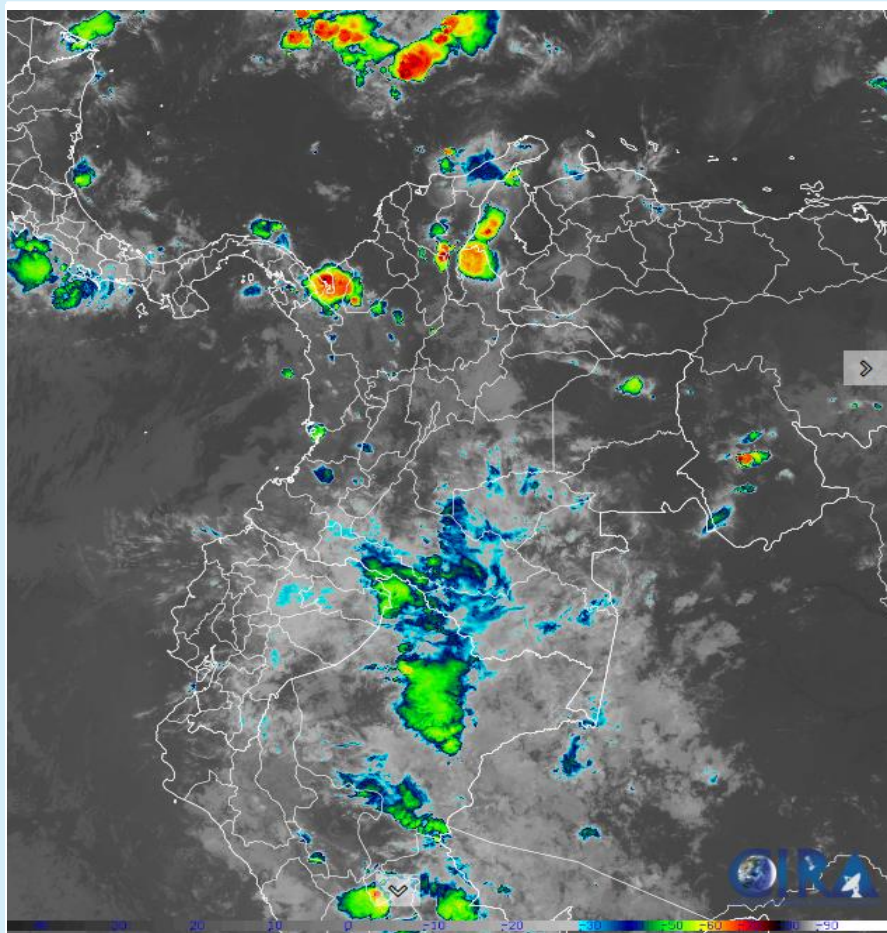
Imagen GOES 16 (East) Canal Infrarrojo | 28 de noviembre de 2024 - Hora 11:00 HLC Fuente: https://rammb-slider.cira.colostate.edu/
