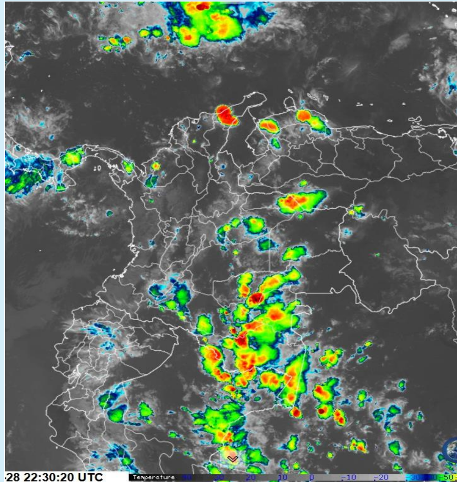
Imagen GOES 16 (East) Canal Infrarrojo | 28 de noviembre de 2024 - Hora 17:30 HLC Fuente: https://rammb-slider.cira.colostate.edu/
