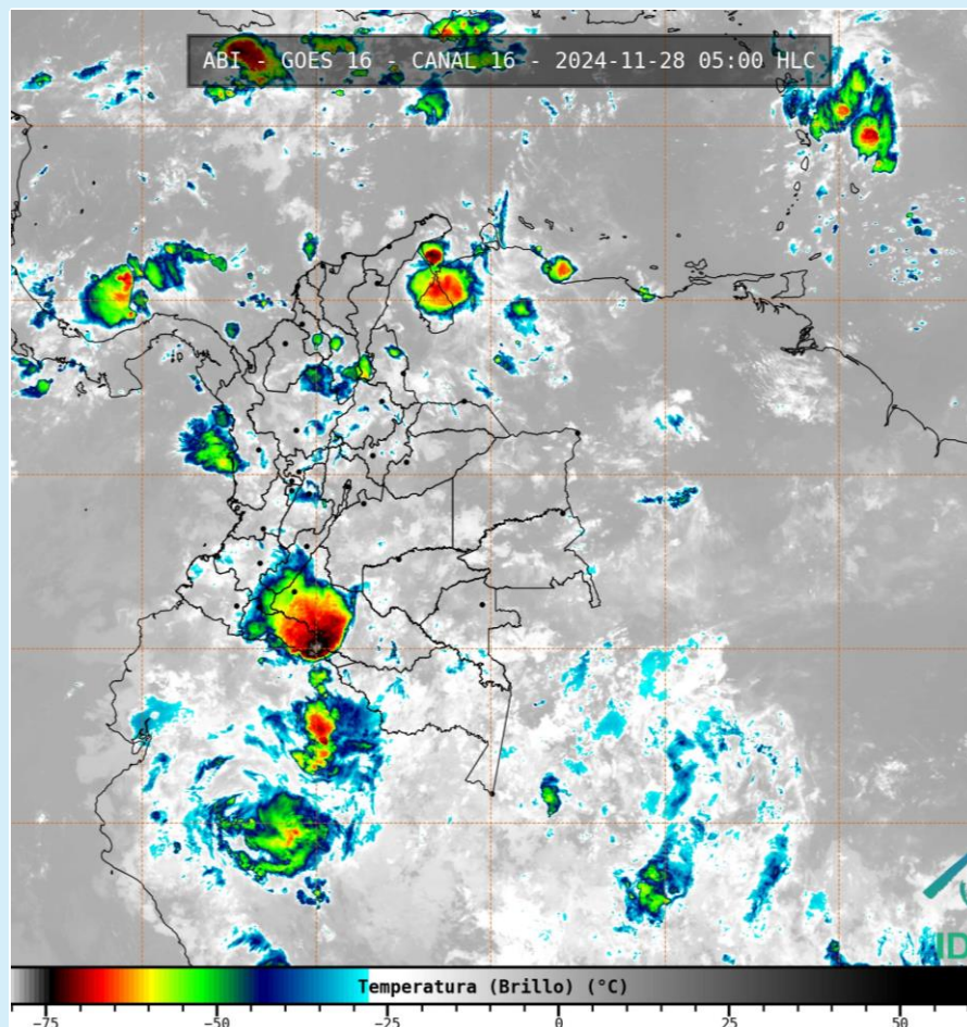
Imagen GOES 16 (East) Canal Infrarrojo | Fuente: GOES 16 - IDEAM 28 de noviembre de 2024 - Hora 05:00 HLC
